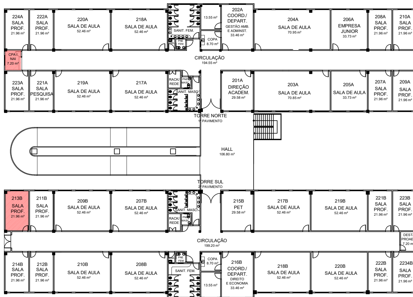
1 PLANTA BAIXA - 2º PAV.
