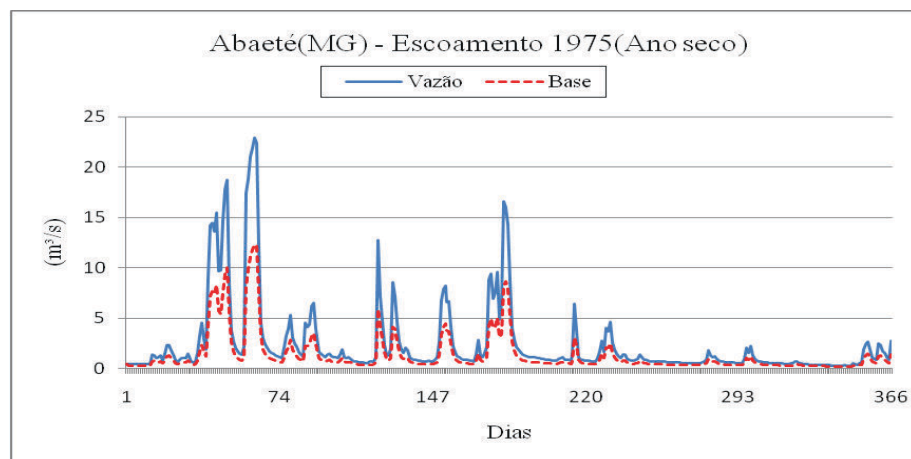
Figura 9. Vazão e escoamento de base do Ribeirão Marmelada em 1975 – Est. Abaeté.
