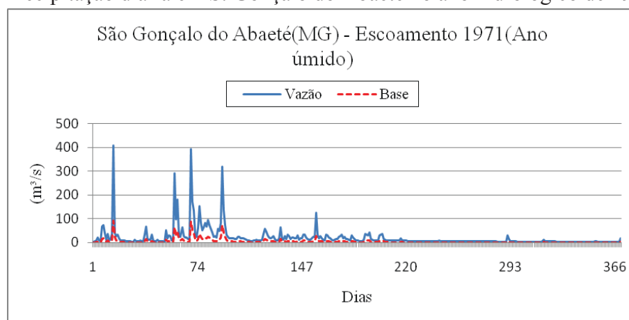
Figura 19. Vazão e escoamento de base do Rio Borrachudo em 1971 – Est. Faz. São Felix.
