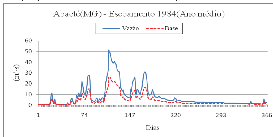
Figura 11. Vazão e escoamento de base do Ribeirão Marmelada em 1984 – Est. Abaeté.
