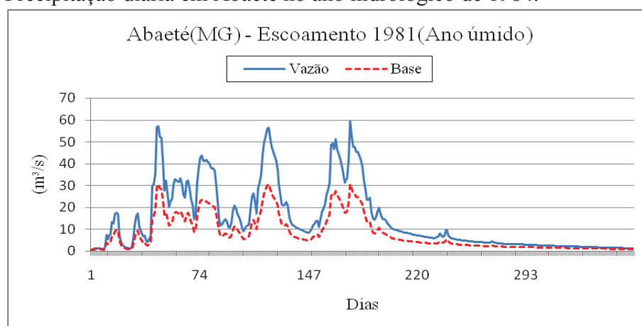
Figura 13. Vazão e escoamento de base do Ribeirão Marmelada em 1981 – Est. Abaeté.
