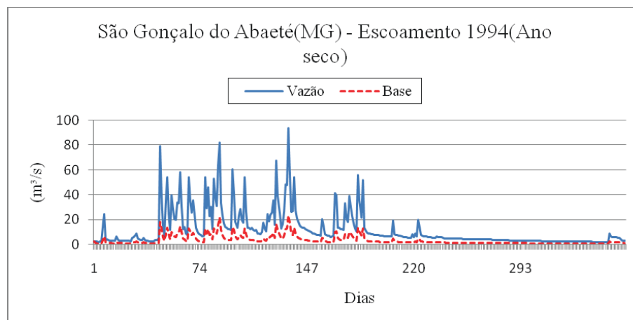
Figura 15. Vazão e escoamento de base do Rio Borrachudo em 1994 – Est. Faz. São Felix.
