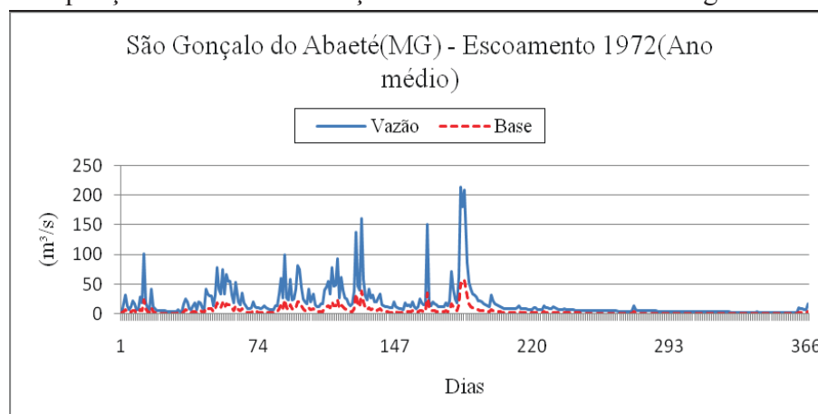
Figura 17. Vazão e escoamento de base do Rio Borrachudo em 1972 – Est. Faz. São Felix.
